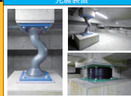
免震装置
